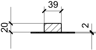
SECTION A-A
