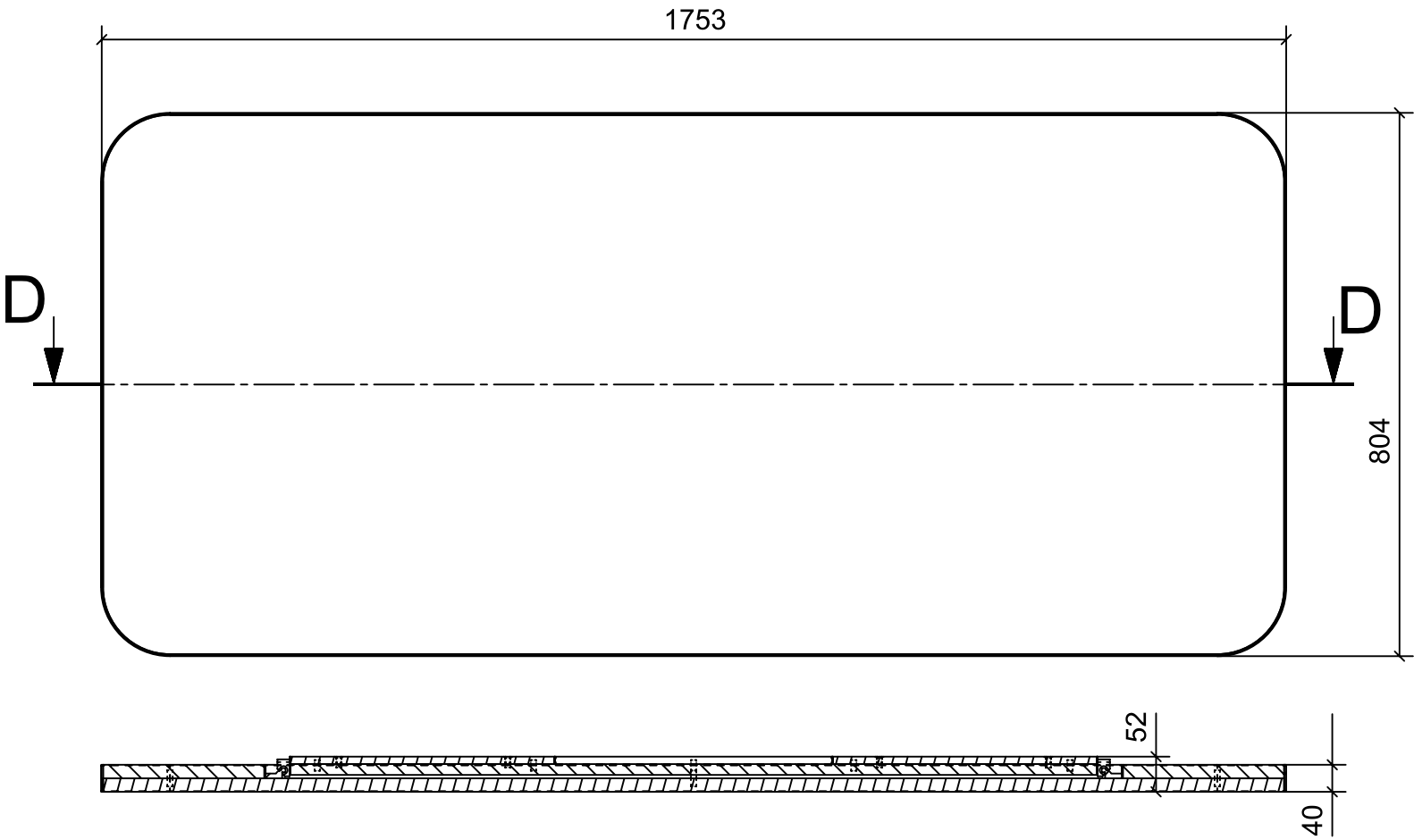
SECTION D-D
