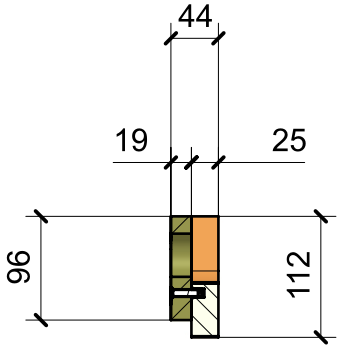
SECTION D-D
