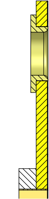
SECTION M-M SCALA 1:2
