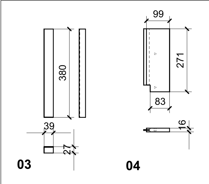
ELEMENTI DA MONTARE in MG_VC02 e spedire con unico imballo
