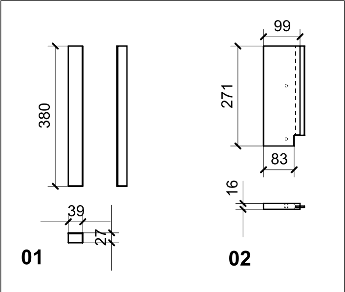
ELEMENTI DA MONTARE in MG_VC01 e spedire con unico imballo
